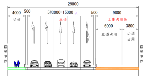
標準断面図
