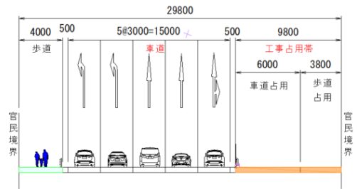
標準断面図
